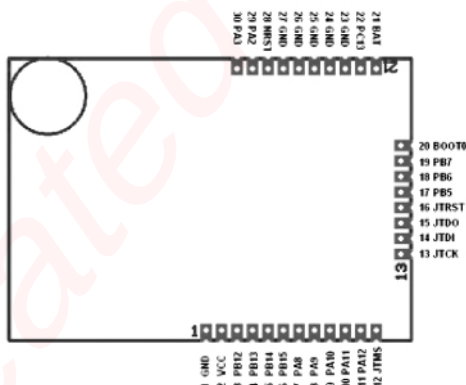
图 2 Z i g b e e 引脚简图
