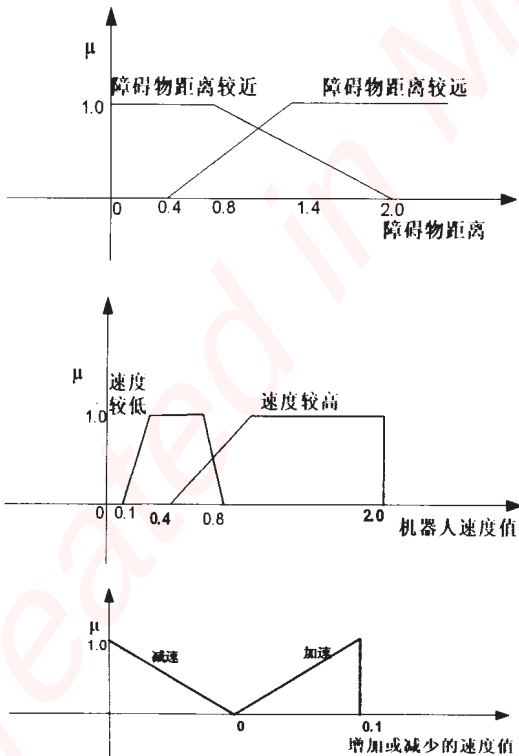
图 5 速度控制隶属函数
