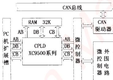
图 1 CAN 通讯卡结构框图
