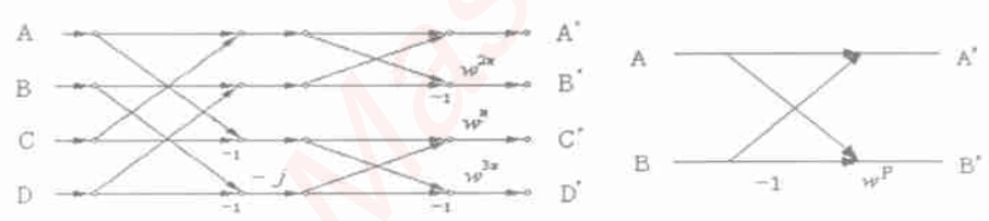
图1 基4-FFT、基2-FFT碟形运算单元
