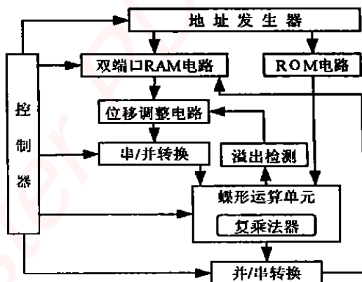
图 2 系统模块图
