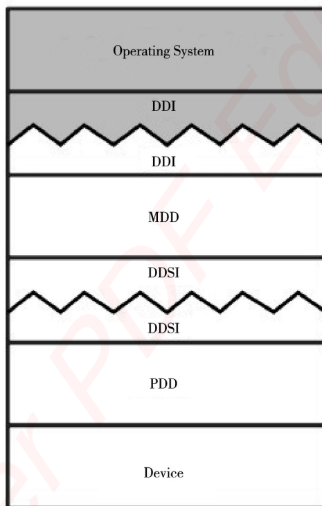
图 1 分层驱动结构图
