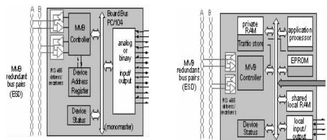
图 2 左图为 MVB I 型网卡结构,右图为 MVB II 型网卡结构
