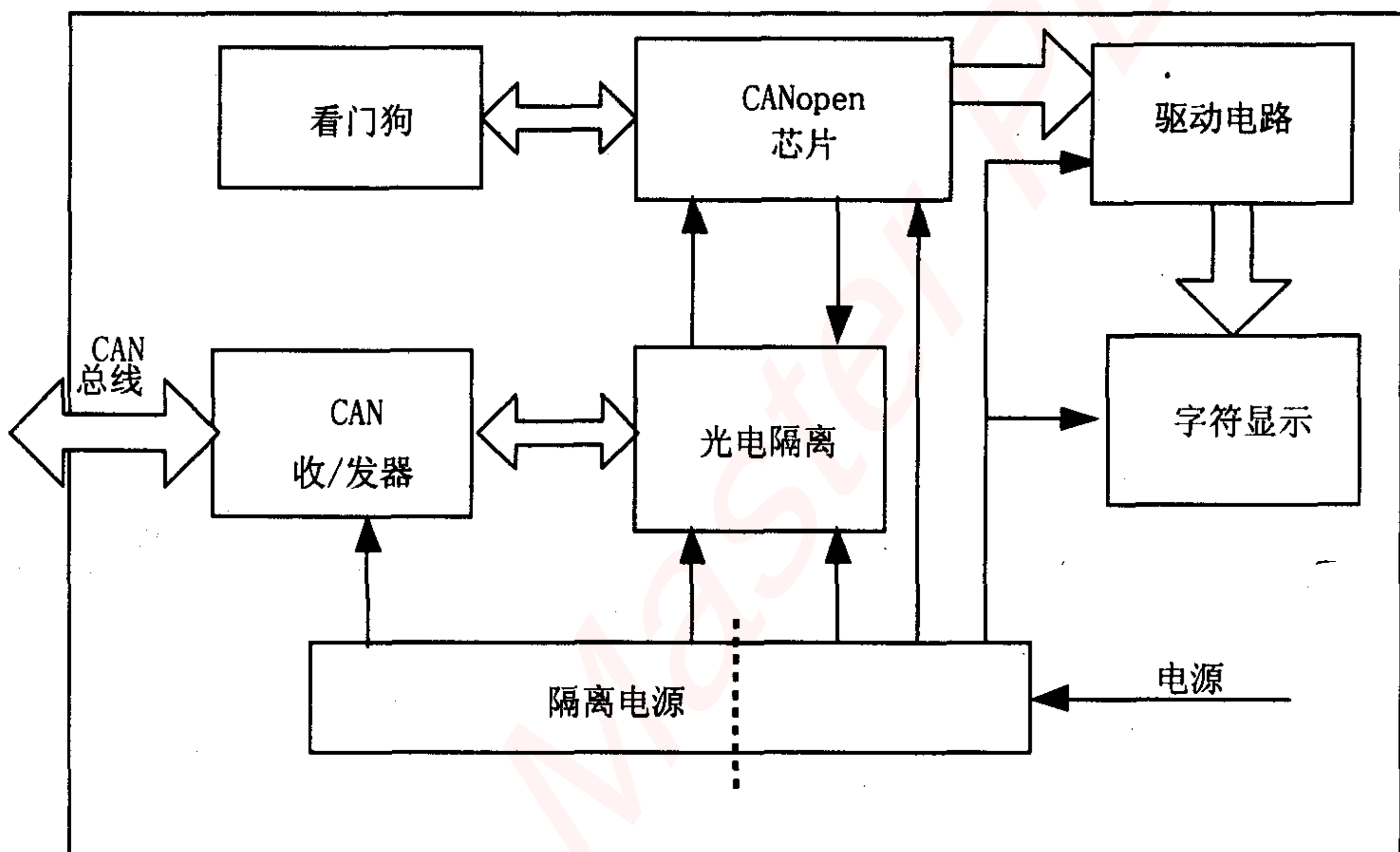
图3 显示 CANopen 节点原理框图
