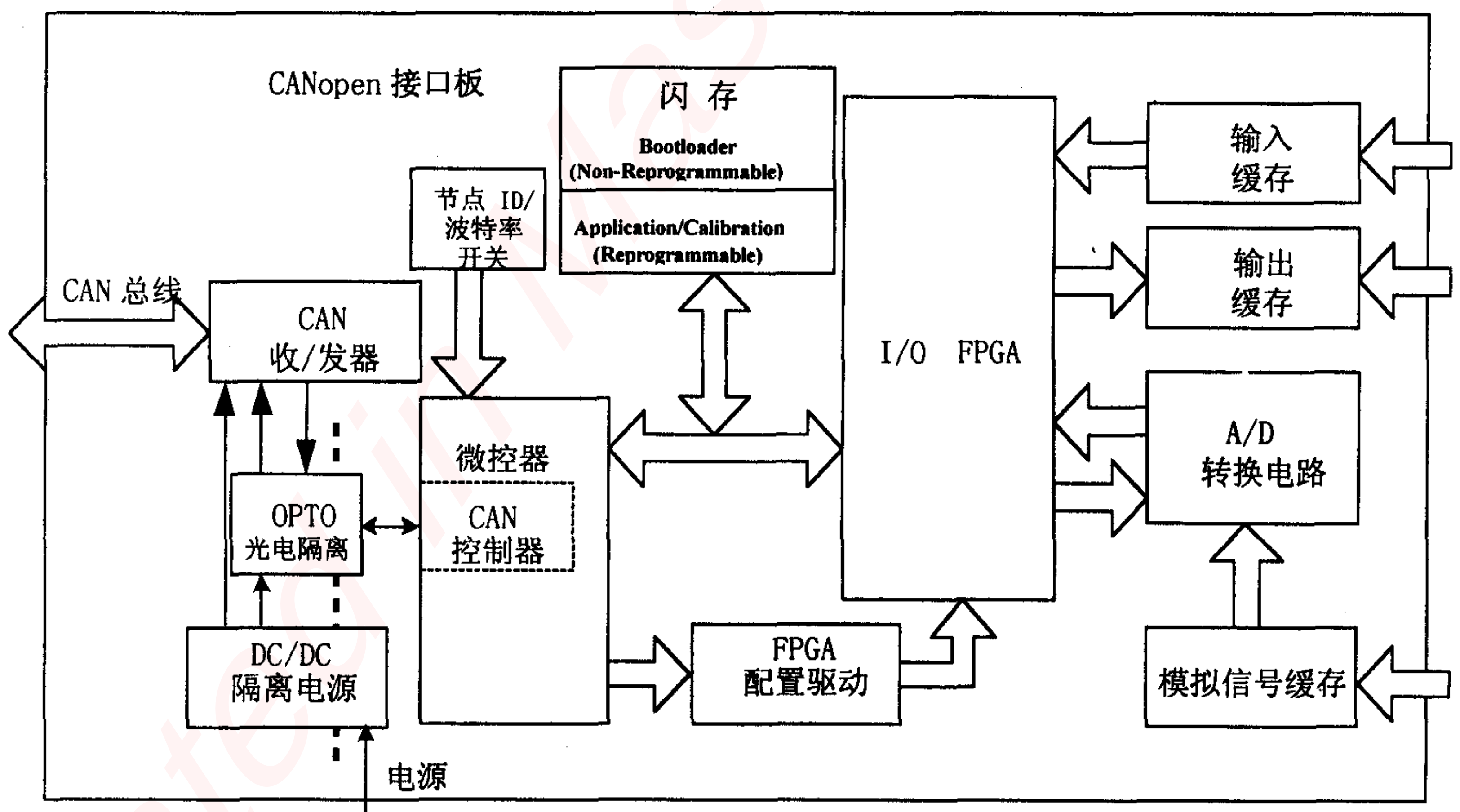
图 2 CANopen 接口板结构图
