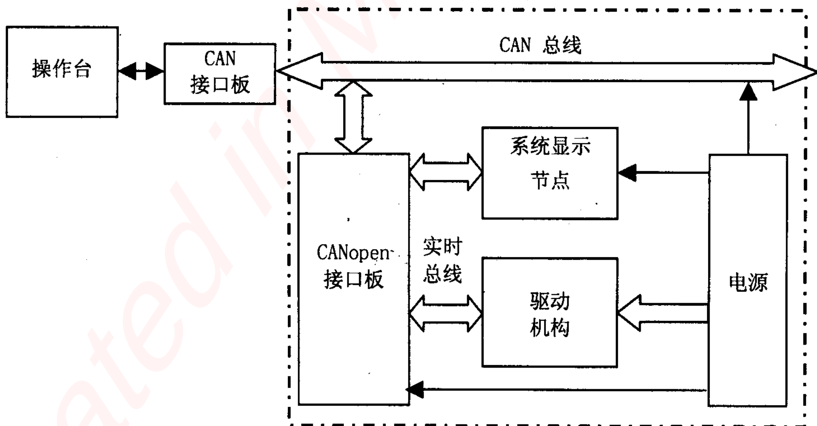
图 1 运动控制单元结构
