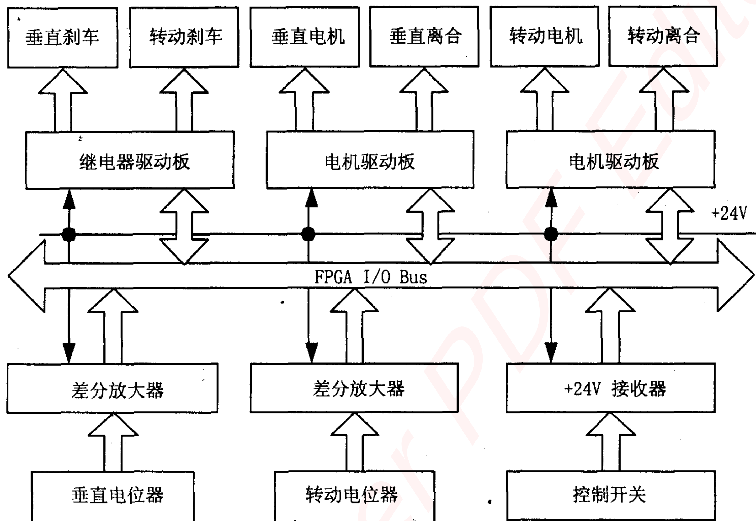
图4 驱动机构原理框图
