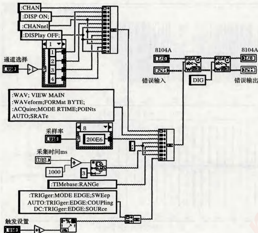
图5 示波器程序原理图
