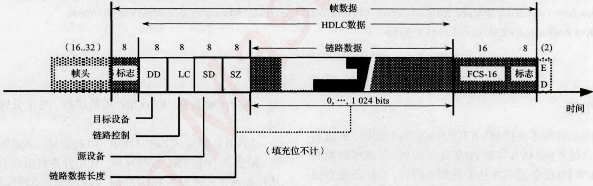
图3 WTB帧
