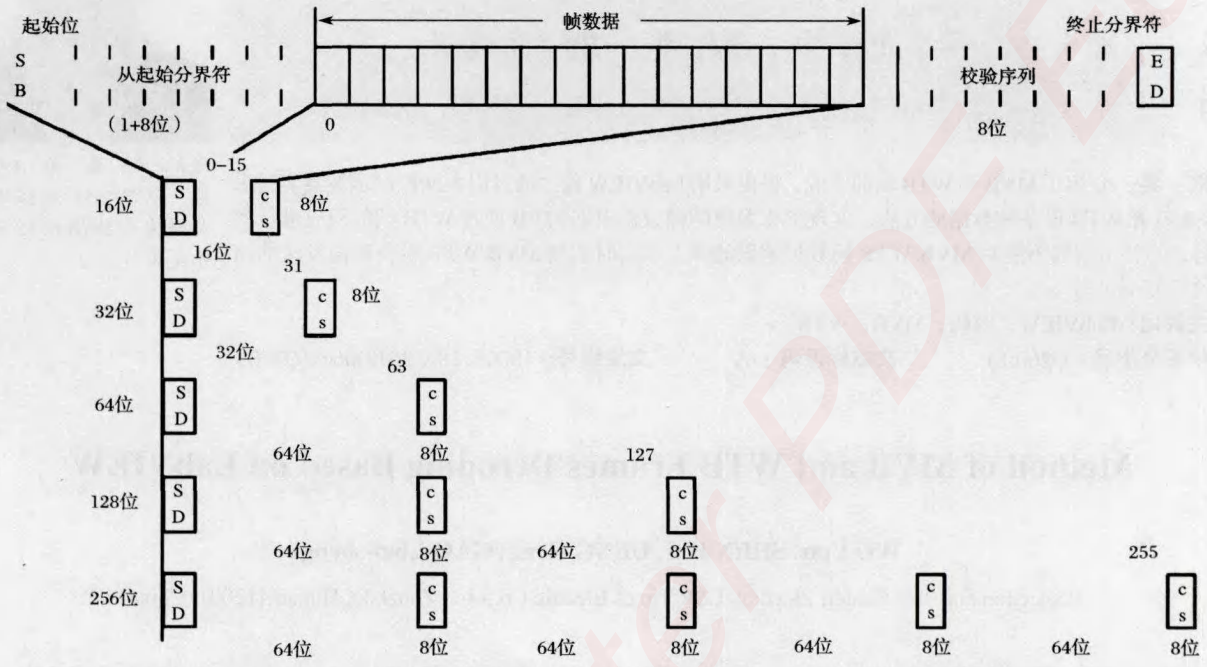
图2 MVB从帧
